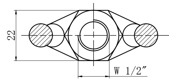
CORTE C-C
